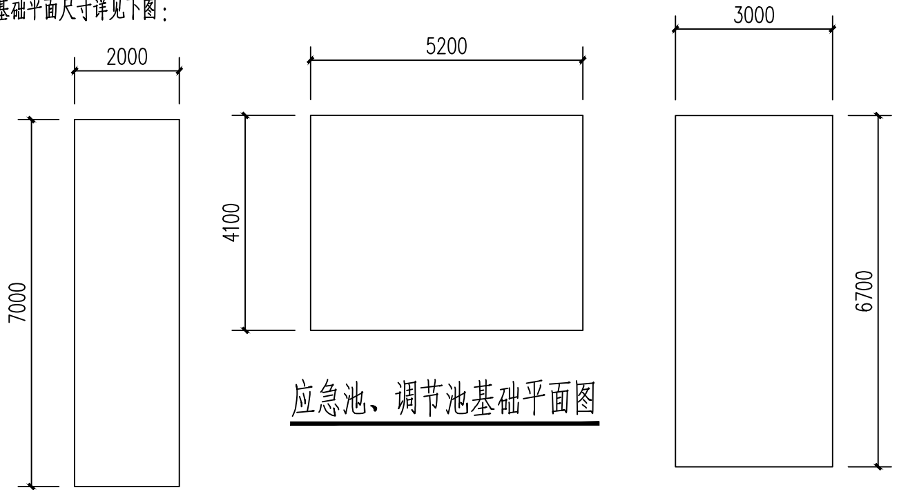
玻璃钢式调节池基础平面图
