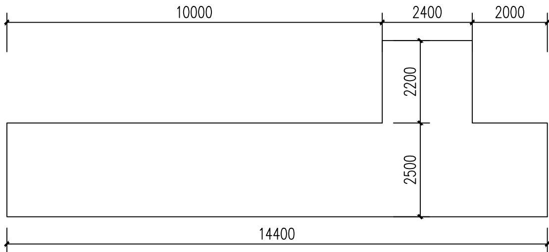
地埋式A2/O一体化设备基础平面图
