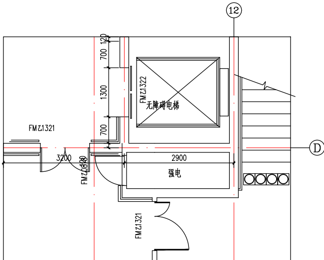
2#楼/4#楼强电井 1:50
