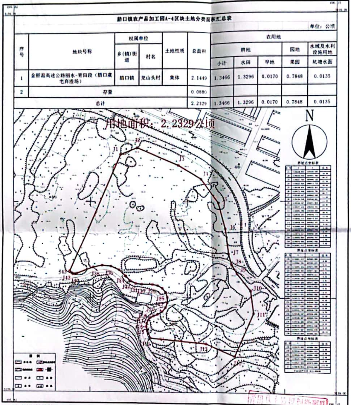
腊口镇农产品加工园A-4区块平面界址图 3139.00-495.82
